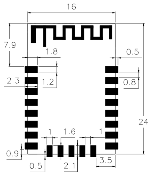
图 7 邮票孔封装尺寸 (单位: mm, 公差±0.1mm, 外围+0.2/-0.1)
