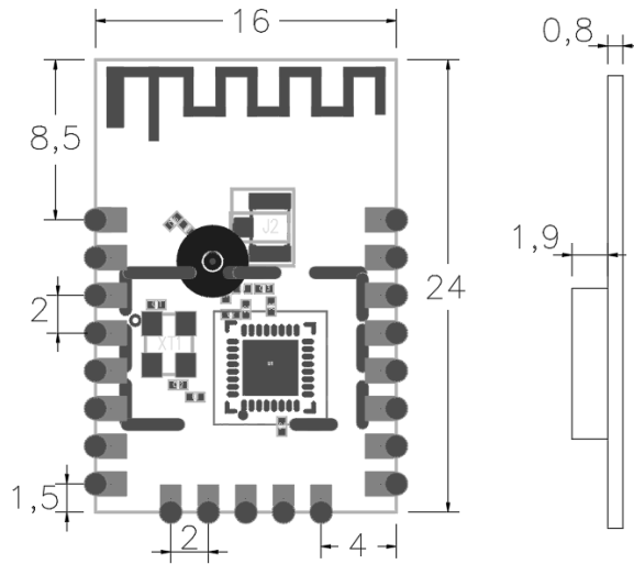
图 6 尺寸图 (单位: mm, 误差±0.1, 外围+0.2/-0.1)
