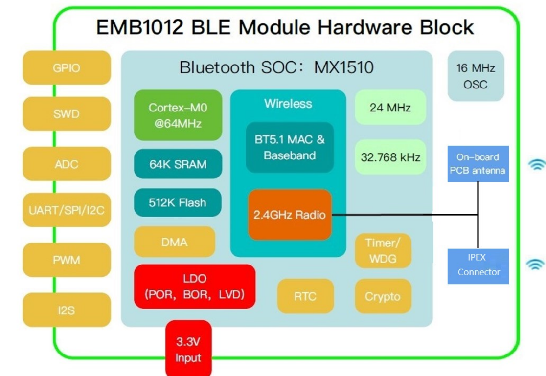
图 1 硬件接口框图
