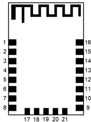
图 2 引脚分布 (俯视图)
