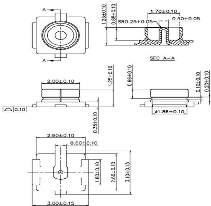
图 5 外接天线连接器尺寸图
