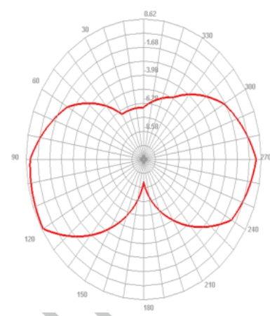
2450.000MHz E2
