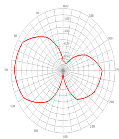
2450.000MHz E1
