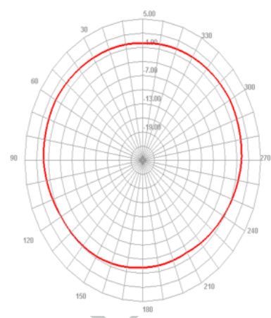
2450.000MHz H
