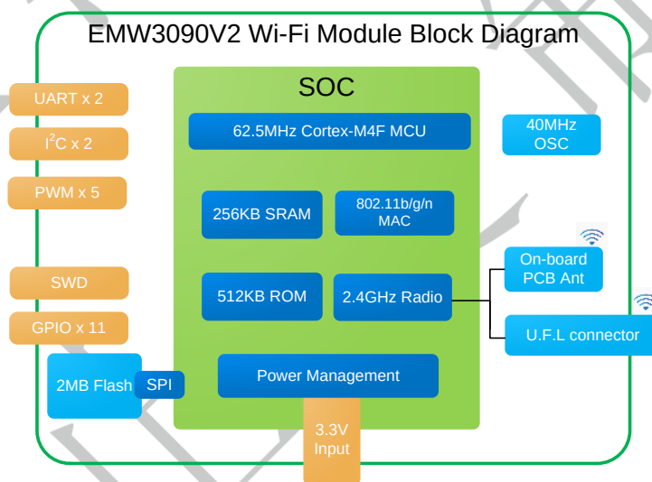
EMW3090V2 硬件框图模块接口
