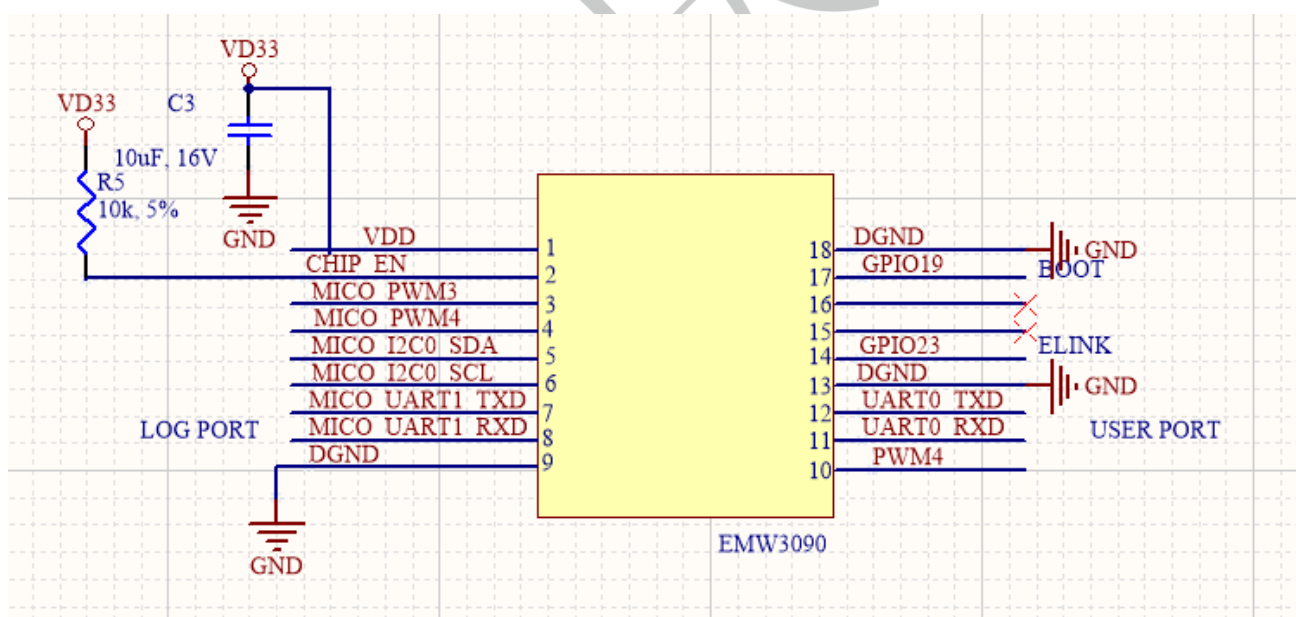
图 11 EMW3090V2 外部接口参考设计
