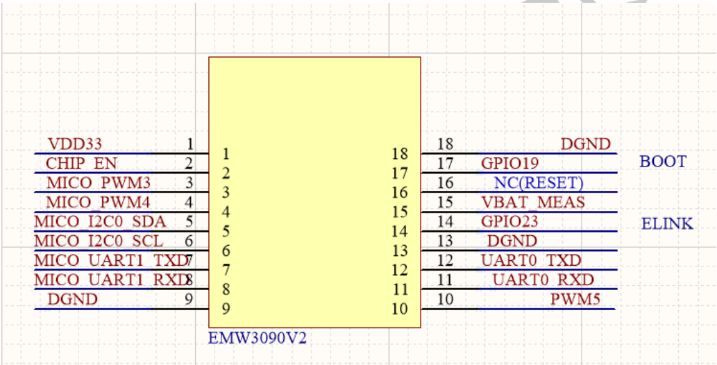
图 3 EMW3090V2 封装定义图
