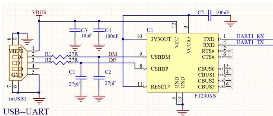
图 10 USB 转串口参考电路
