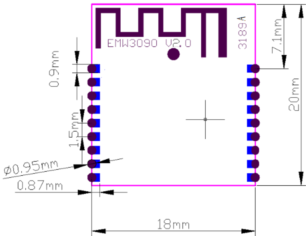
图 2 邮票孔封装尺寸图
