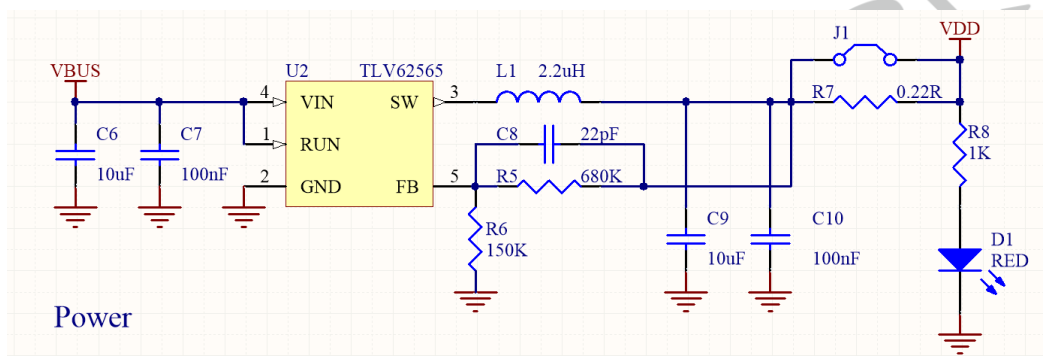
图 9 电源参考电路
