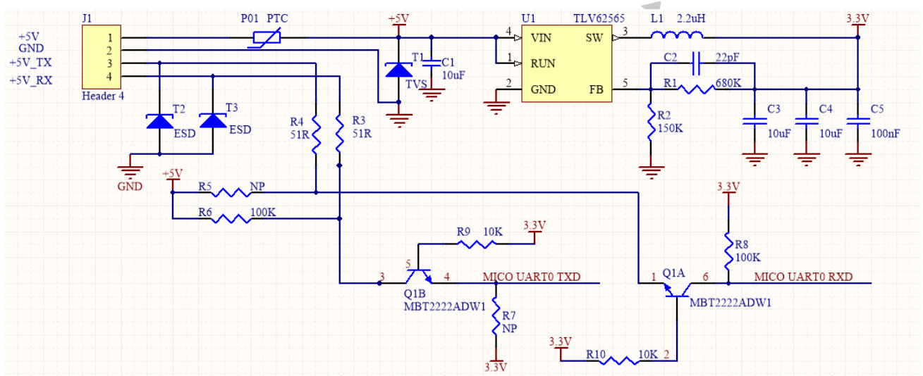
图 12 3.3V UART- 5V UART 转换电路
