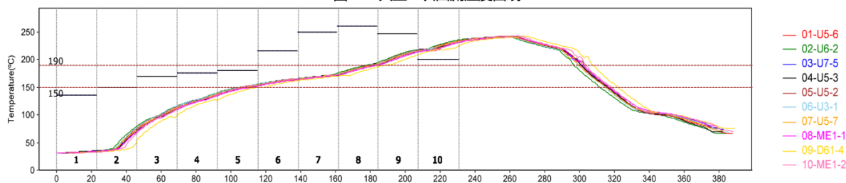
图 14 典型二次回流温度曲线
