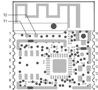
图 2 引脚分布
