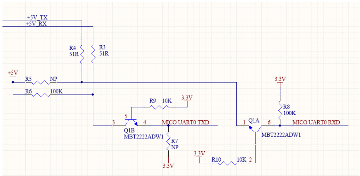
图 12 UART 3.3V/5V转换电路
