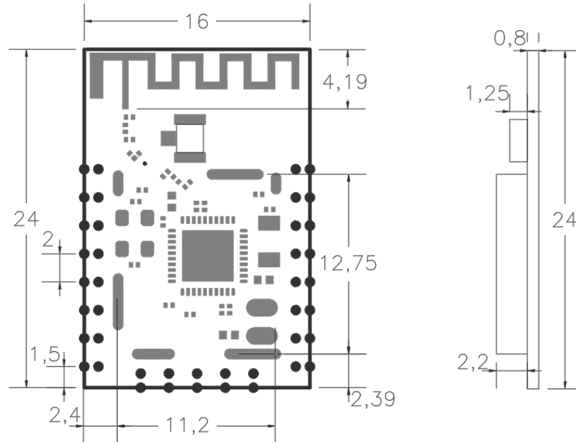
图 6 尺寸图 (单位: mm, 误差±0.1, 外围+0.2/-0.1)
