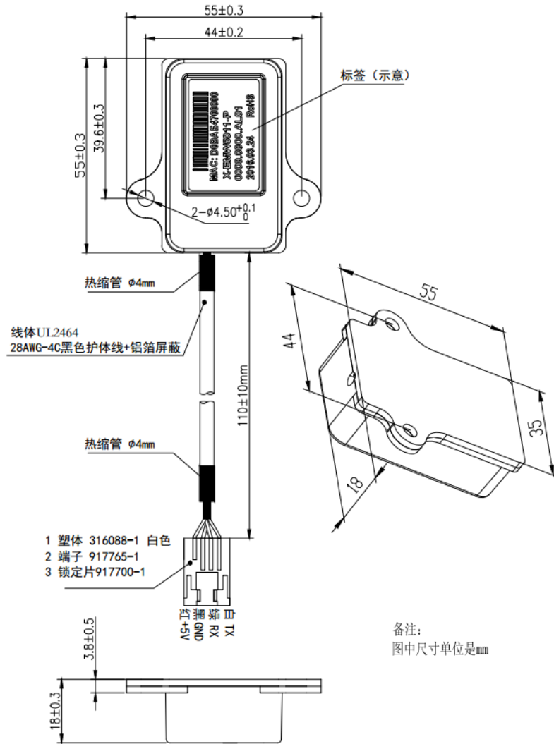
图 16 灌胶盒尺寸图 (单位: mm)
