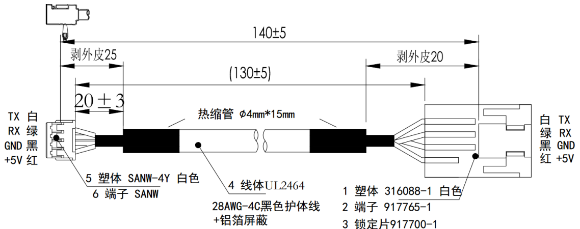
图 17 灌胶盒线束尺寸图 (单位: mm)
