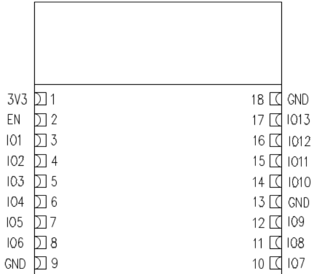
图 2 引脚分布
